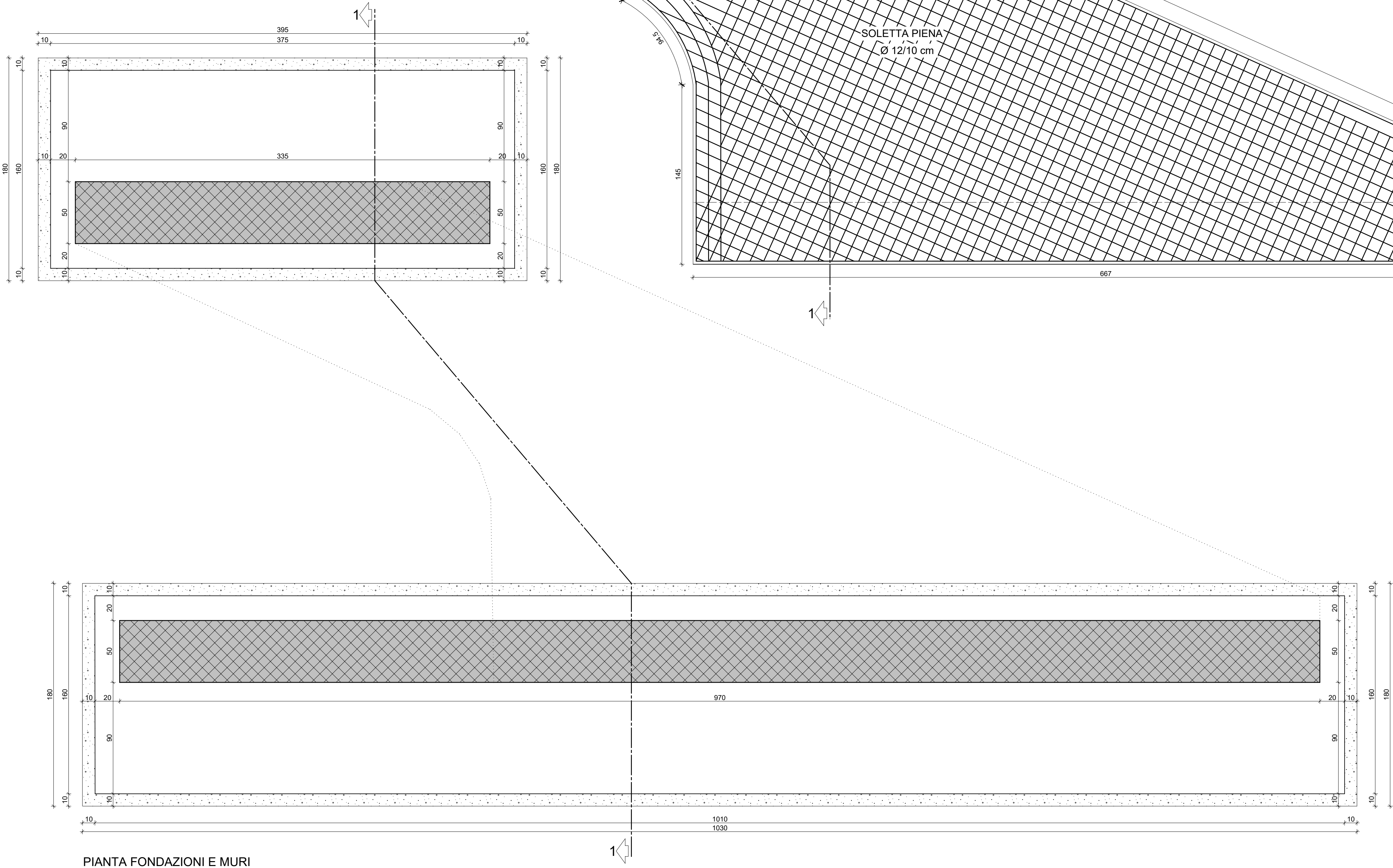
PIANTA FONDAZIONI E MURI
